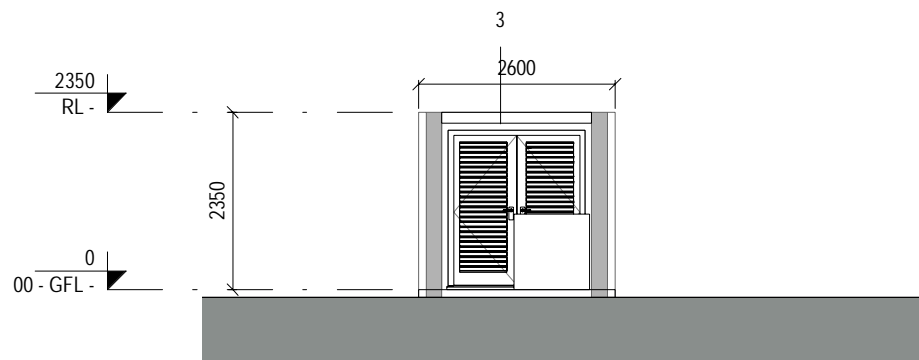
8 Section A-A 1 : 100
